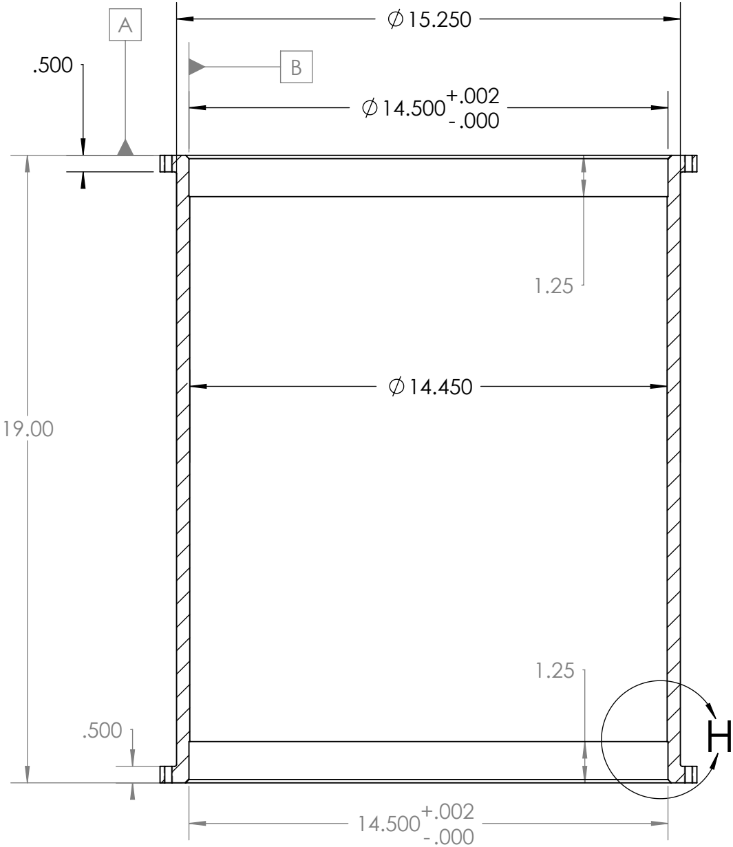
SECTION G-G SCALE 1 : 4
