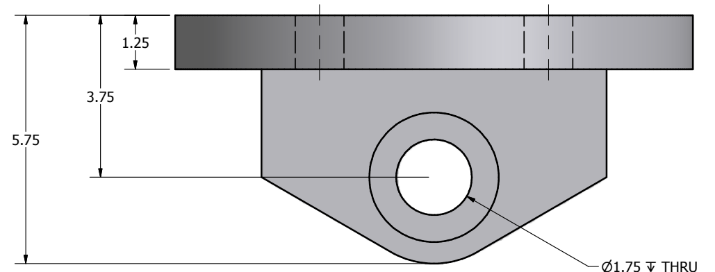
VIEW A-A
