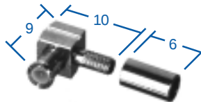
FIG. 2 RMX-8010-A, -B, -B1, -1B
