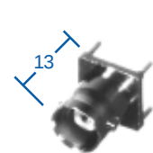
FIG. 35 RFB-1115-11
