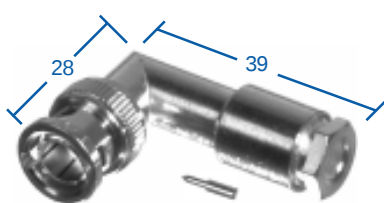
FIG. 7 RFB-1709-D
