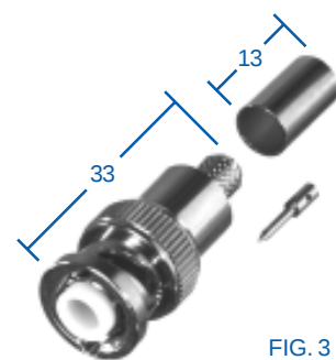
FIG. 3 RHV-106-D
