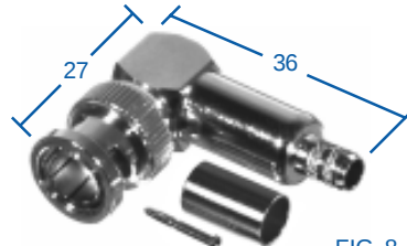
FIG. 8 RFB-1710-D, -J, -K, -W
