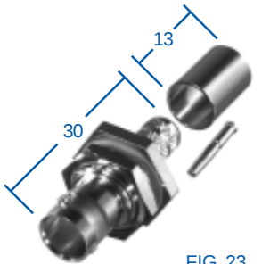
FIG. 23 RFB-1717-Q
