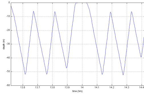
Fig. 15. Glider depth profiles (zoom).
