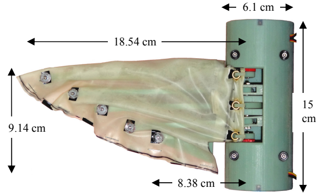
Fig. 5. The Gen2 fin.
