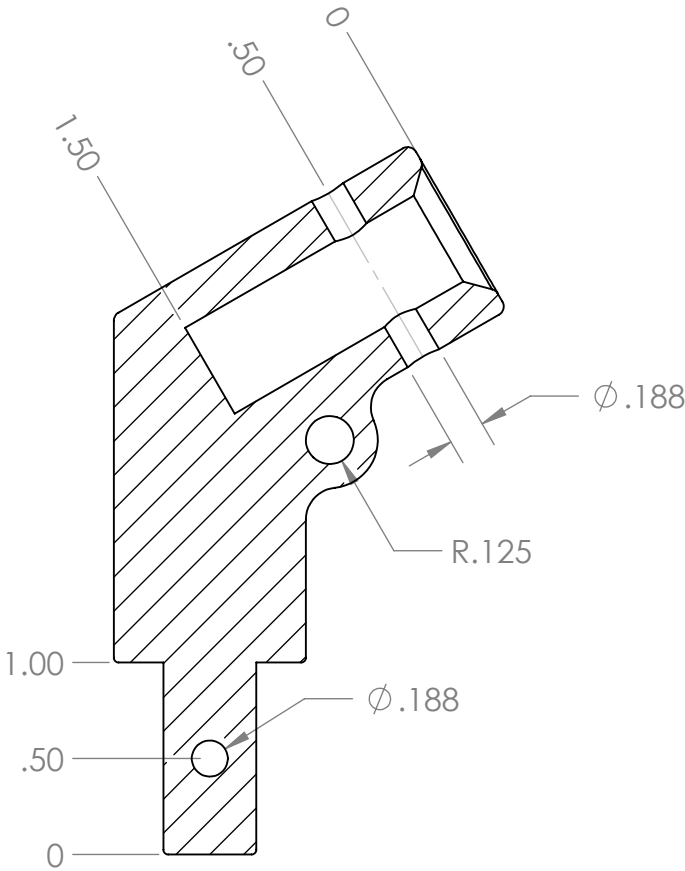
SECTION A-A
