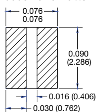
0508 Land Pattern
