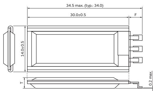
DMF4B5R5G105M3DTA0
