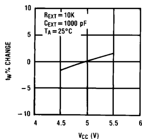
DM9602
