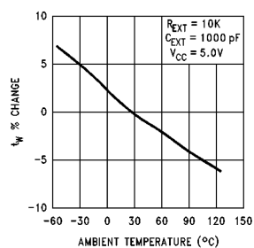
DM9602
