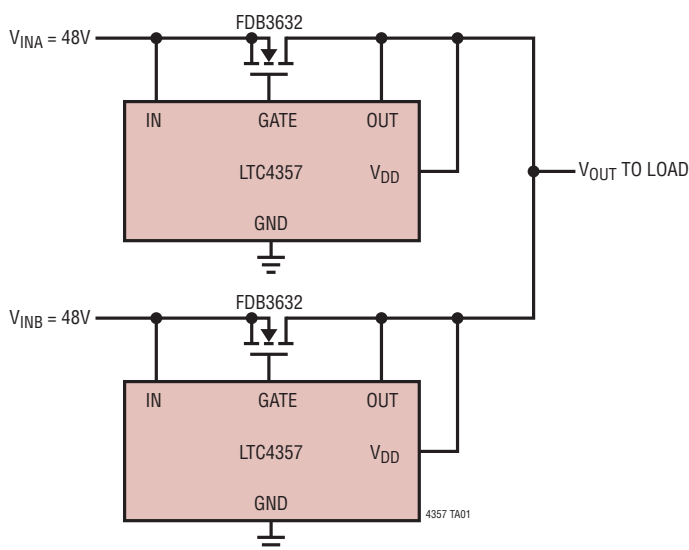
48V, 10A Diode-OR
