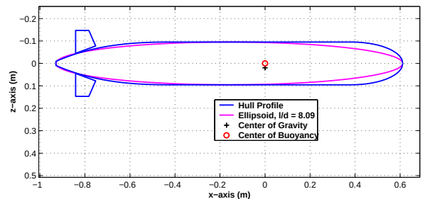
Fig. 1: REMUS Profile (XZ-plane)
