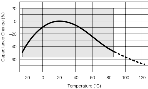
Char. E/Y5U
