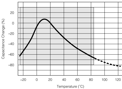
Char. F/Y5V
