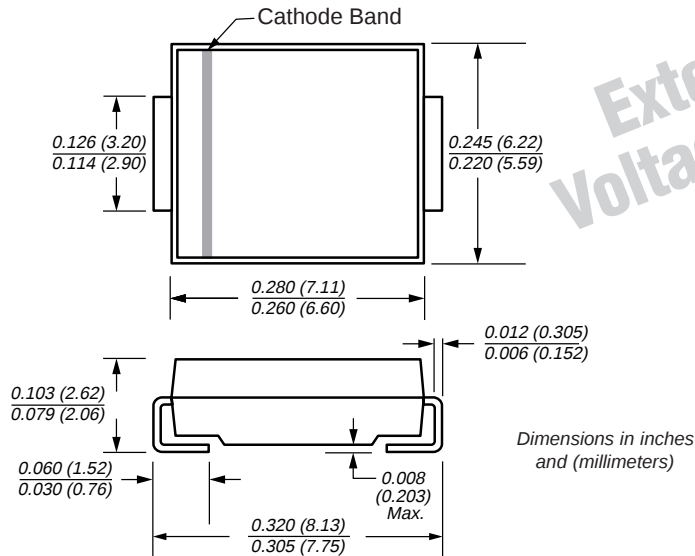
DO-214AB (SMC J-Bend)
