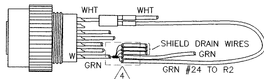
SHIELD DRAIN WIRING TYP.
