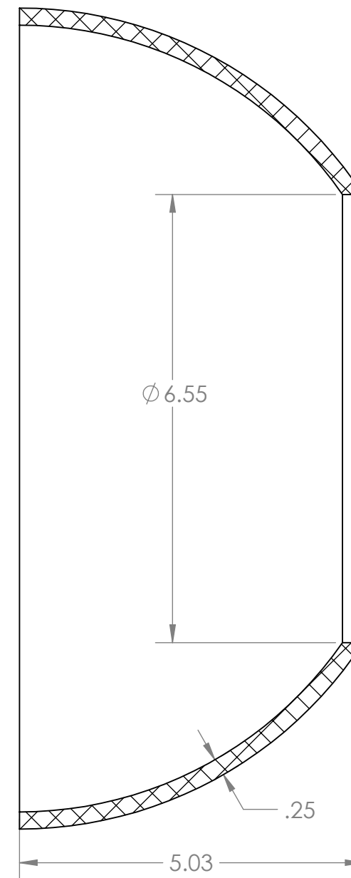
SECTION B-B SCALE 1 : 2
