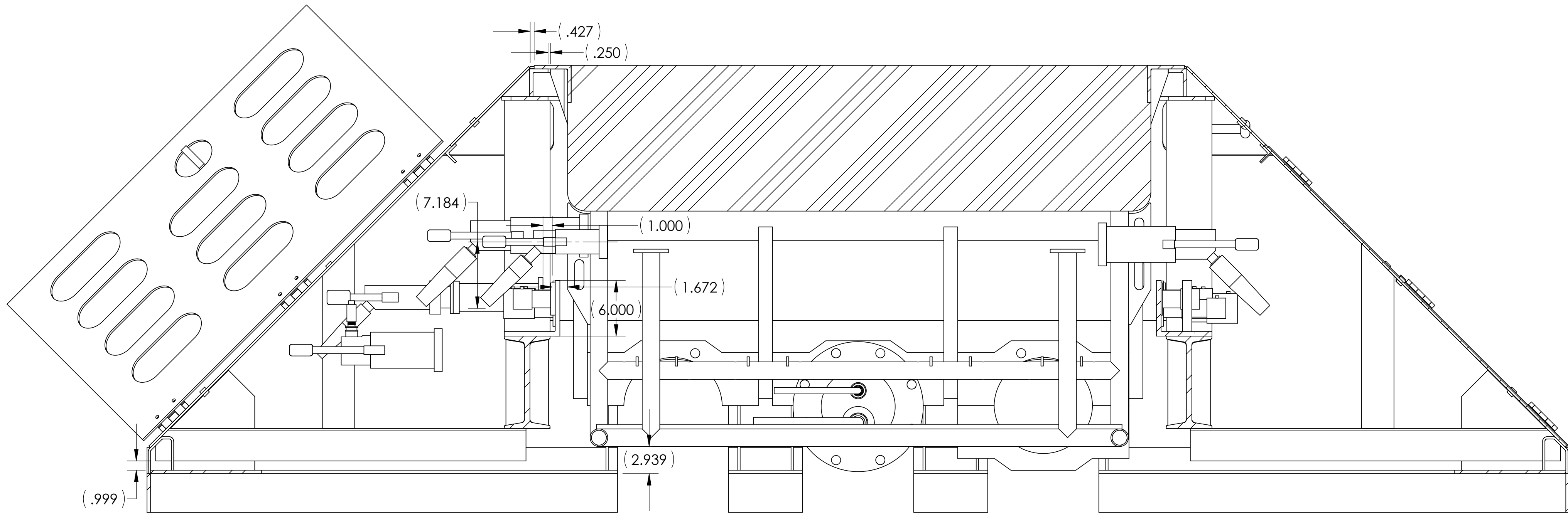
SECTION A-A SCALE 1 : 8
