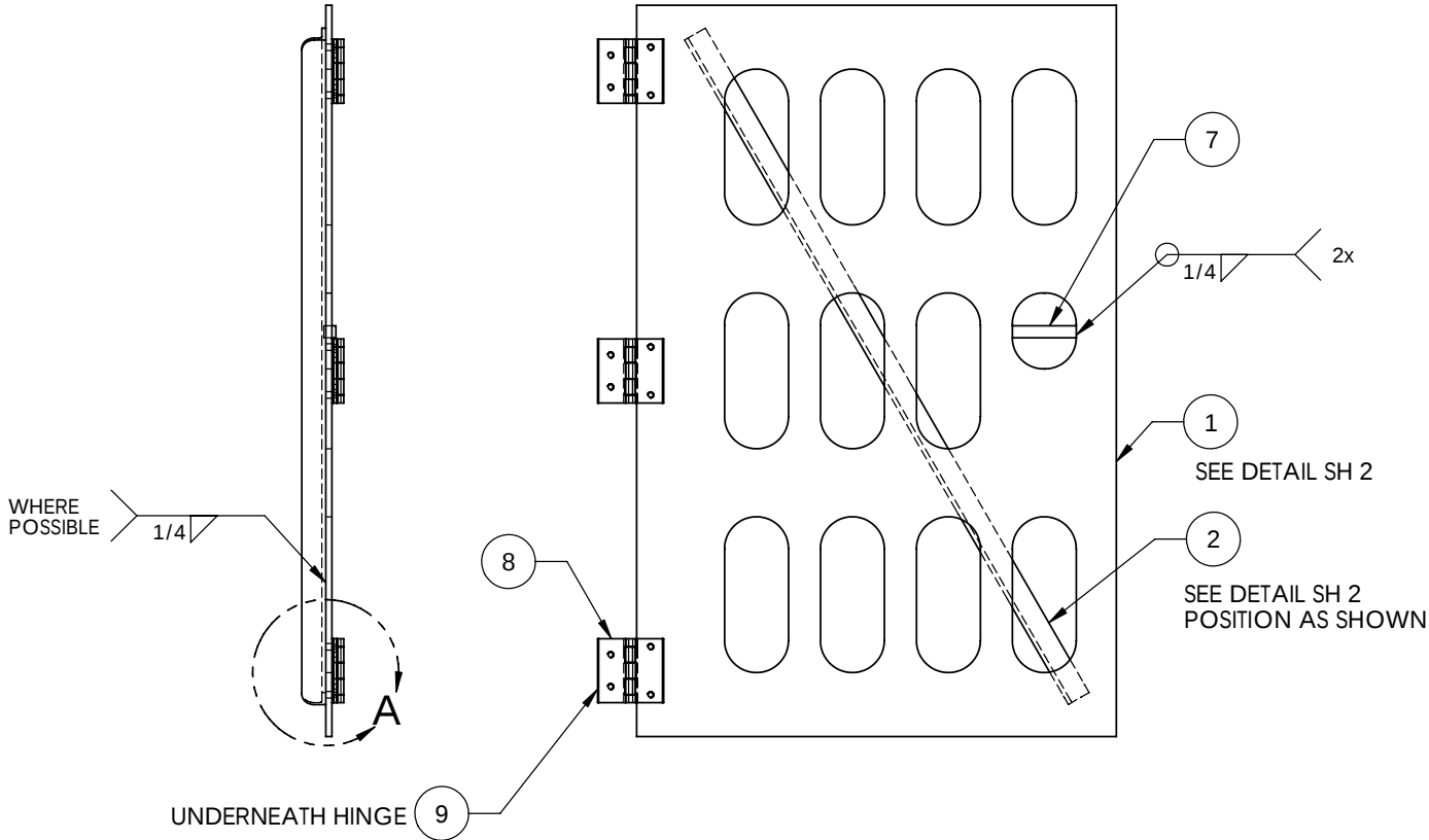
110434-54 DOOR ASSEMBLY, LEFT
