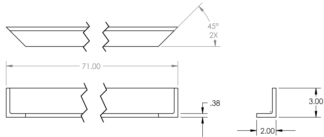
2 110434-97 MATERIAL: A-36 L 3 X 2 X 3/8 REQ'D:2
