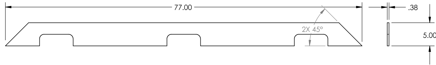
4 110434-94 MATERIAL: A-36 3/8 X 5 REQ'D:2
