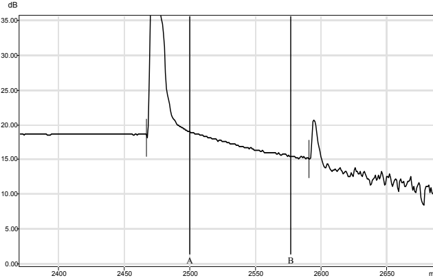
CTA-ODIsde-fiber6.trc (1550 nm)
