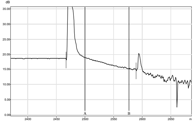
CTA-ODIsde-fiber7.trc (1550 nm)
