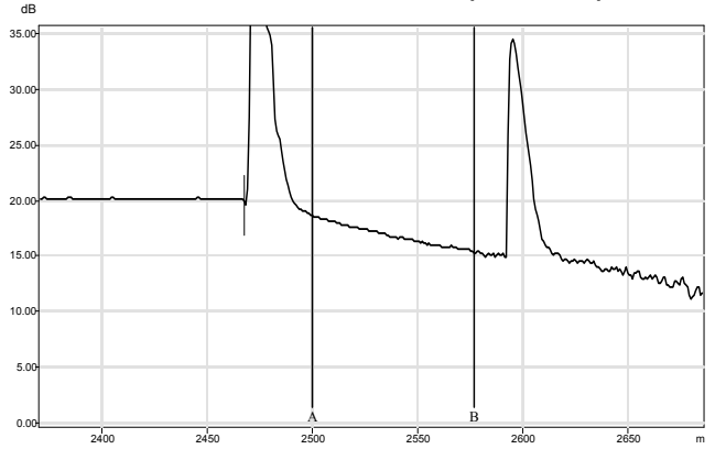
CTA-ODIsde-fiber1.trc (1310 nm)
