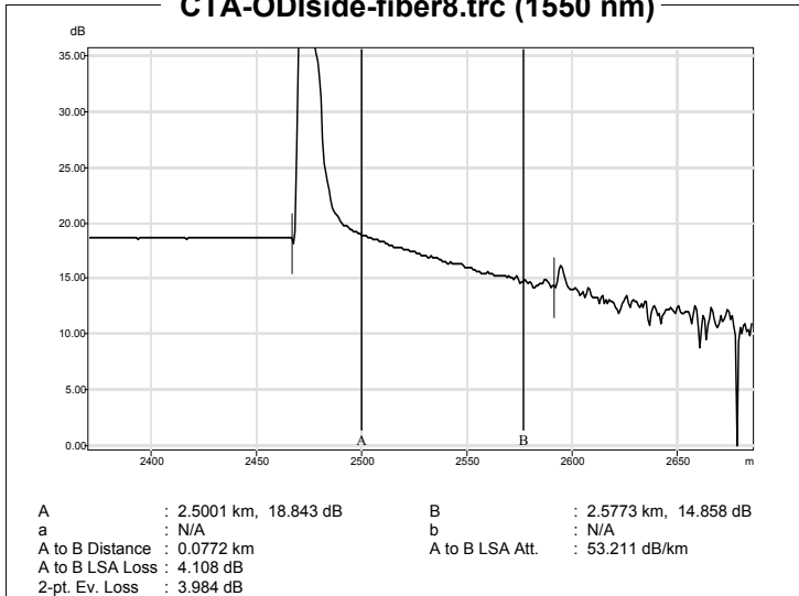
CTA-ODIside-fiber8.trc (1550 nm)
