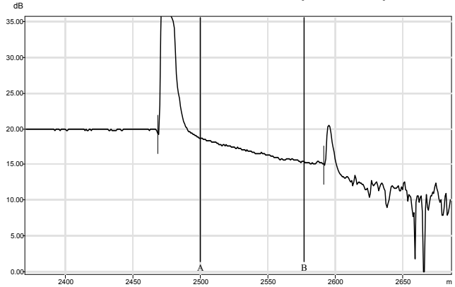
CTA-ODIsde-fiber7.trc (1310 nm)
