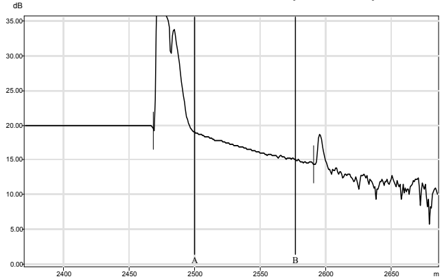
CTA-ODIside-fiber5.trc (1310 nm)
