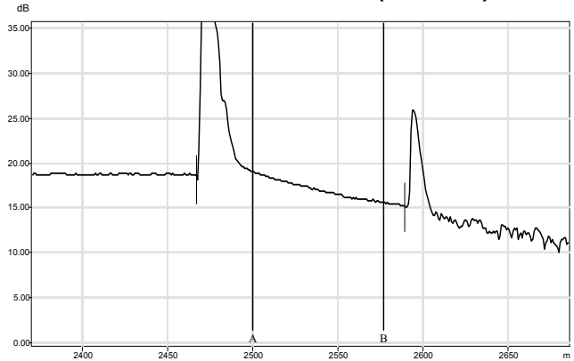
CTA-ODIside-fiber3.trc (1550 nm)
