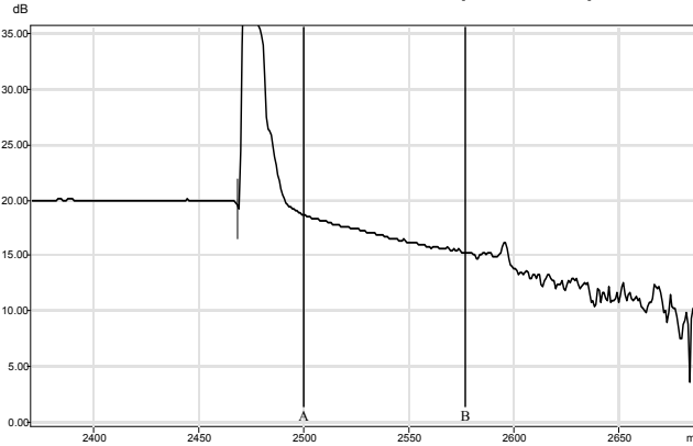
CTA-ODIside-fiber4.trc (1310 nm)
