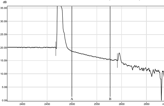
CTA-ODIside-fiber2.trc (1310 nm)
