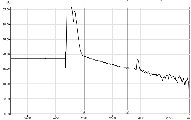
CTA-ODIside-fiber5.trc (1550 nm)
