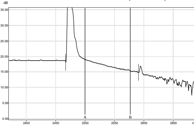
CTA-ODIside-fiber4.trc (1550 nm)
