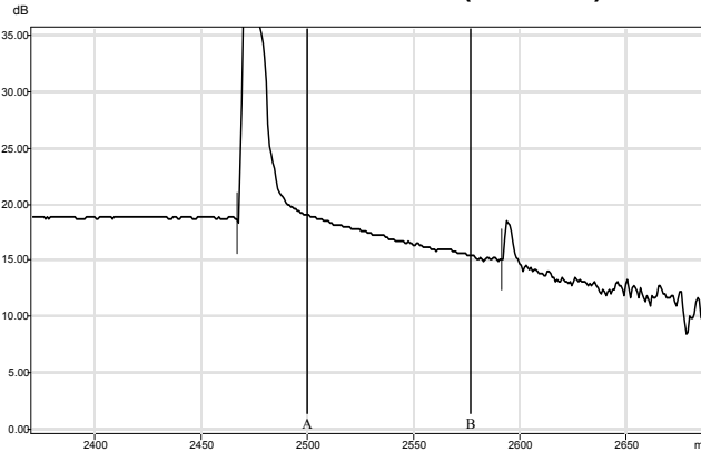
CTA-ODIside-fiber2.trc (1550 nm)
