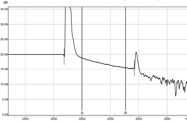
CTA-ODIsde-fiber6.trc (1310 nm)
