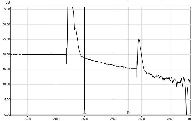
CTA-ODIside-fiber3.trc (1310 nm)
