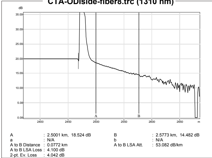
CTA-ODIside-fiber8.trc (1310 nm)
