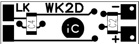
BOTTOM
