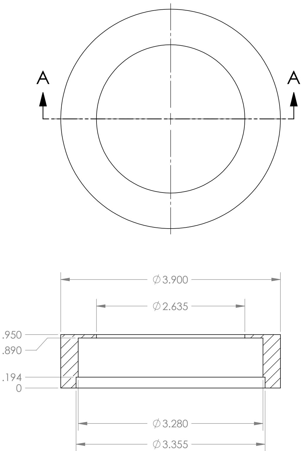
SECTION A-A
