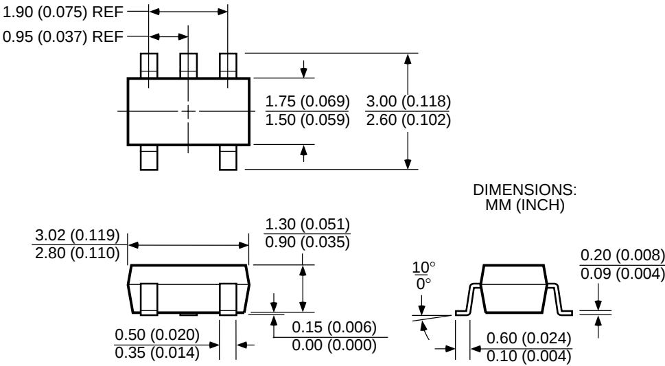
SOT-23-5 (M5)
