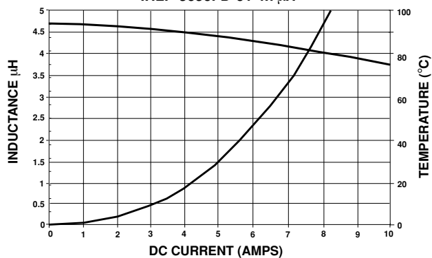
IHLP-5050FD-01 4.7 \mu H
