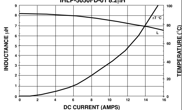
IHLP-5050FD-01 8.2 \mu H
