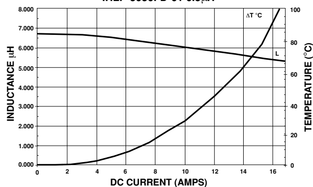
IHLP-5050FD-01 6.8 \mu H
