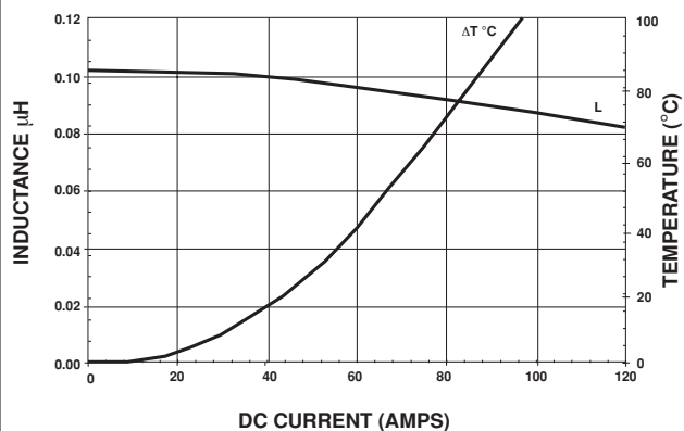
IHLP-5050FD-01 0.10 \mu H
