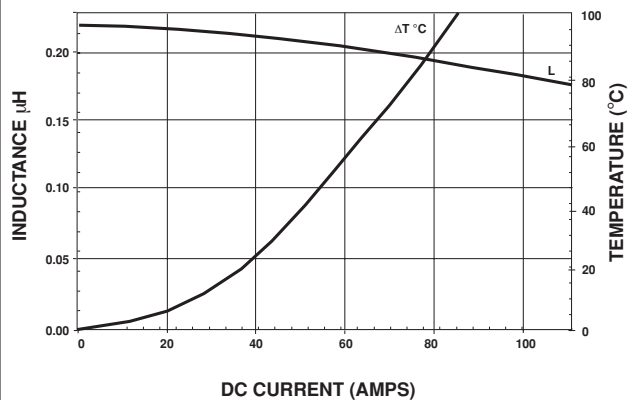
IHLP-5050FD-01 0.22 \mu H
