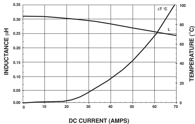
IHLP-5050FD-01 0.30 \mu H
