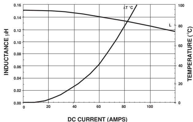
IHLP-5050FD-01 0.15 \mu H
