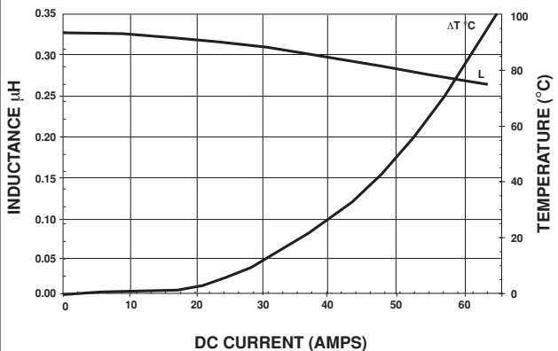
IHLP-5050FD-01 0.33 \mu H
