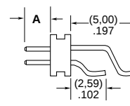
-DH OPTION
