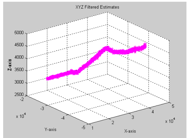
Fig. 7. Target 2 Trajectory
