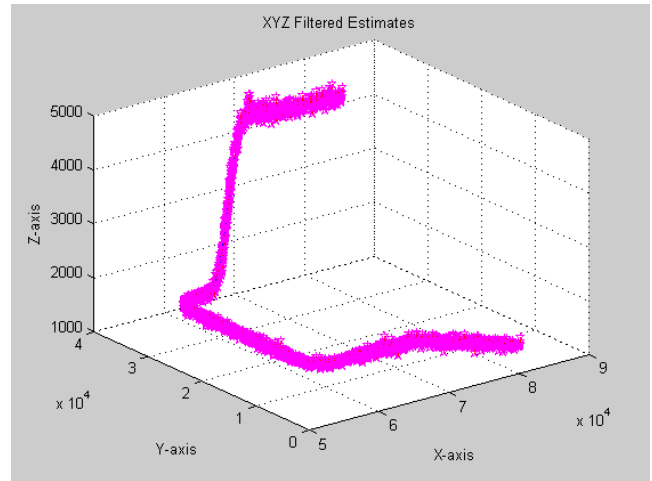
Fig. 20. Target 5 Trajectory
