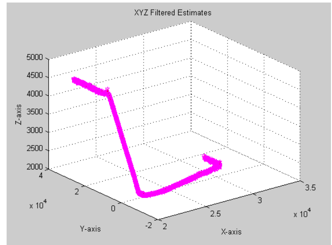
Fig. 15. Target 4 Trajectory
