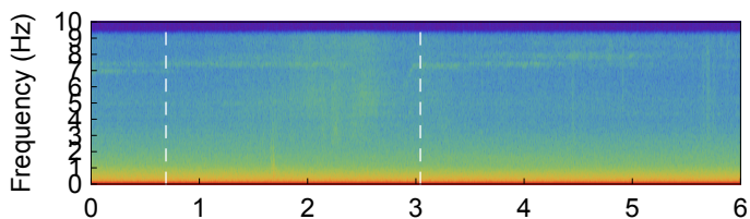
MOBB Seismometer EW Axis
