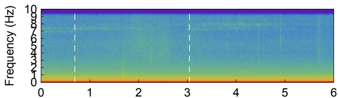
MOBB Seismometer NS Axis
