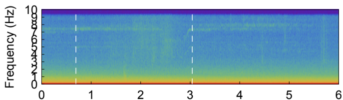
MOBB Seismometer Z Axis
