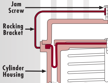
Fig. 26: Pivot Rocking Bracket
