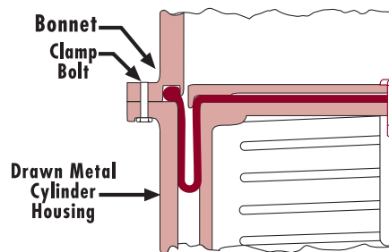
Fig. 30: Grooved Bonnet
