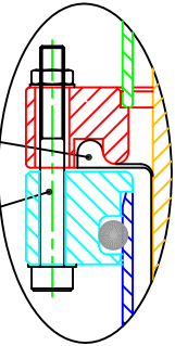
SECTION B-B TYP 12 POS' 9 13 14 15 2
