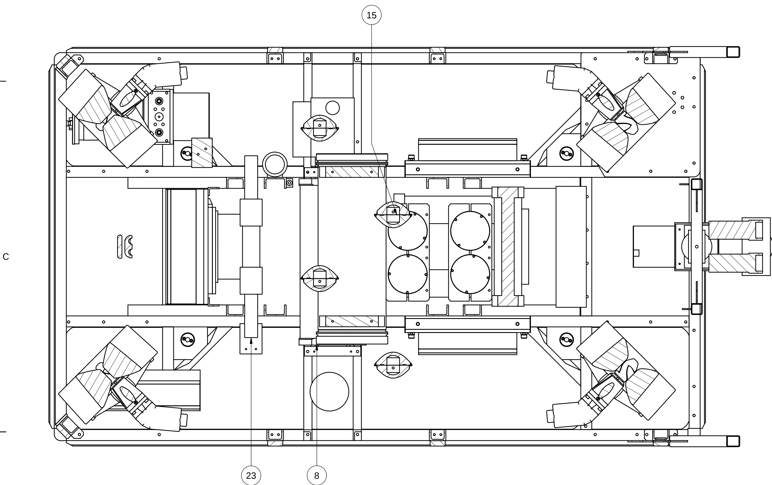
SECTION A-A
