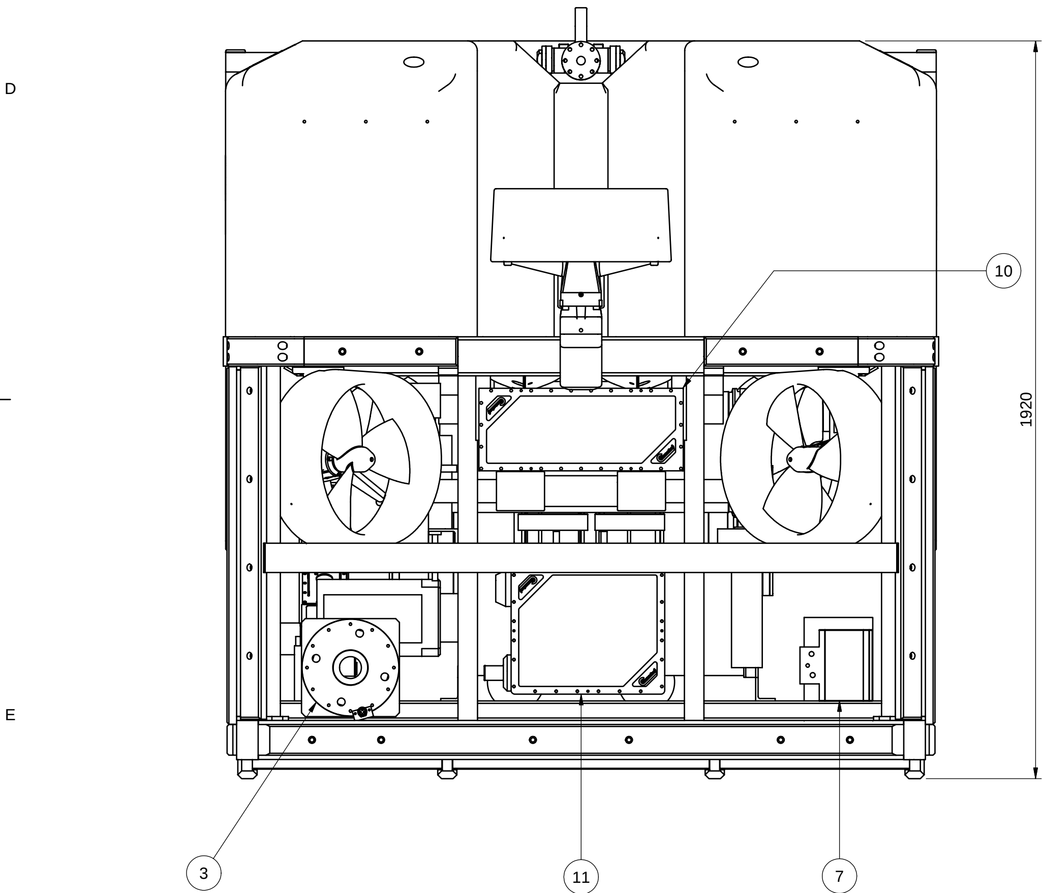
SECTION A-A
