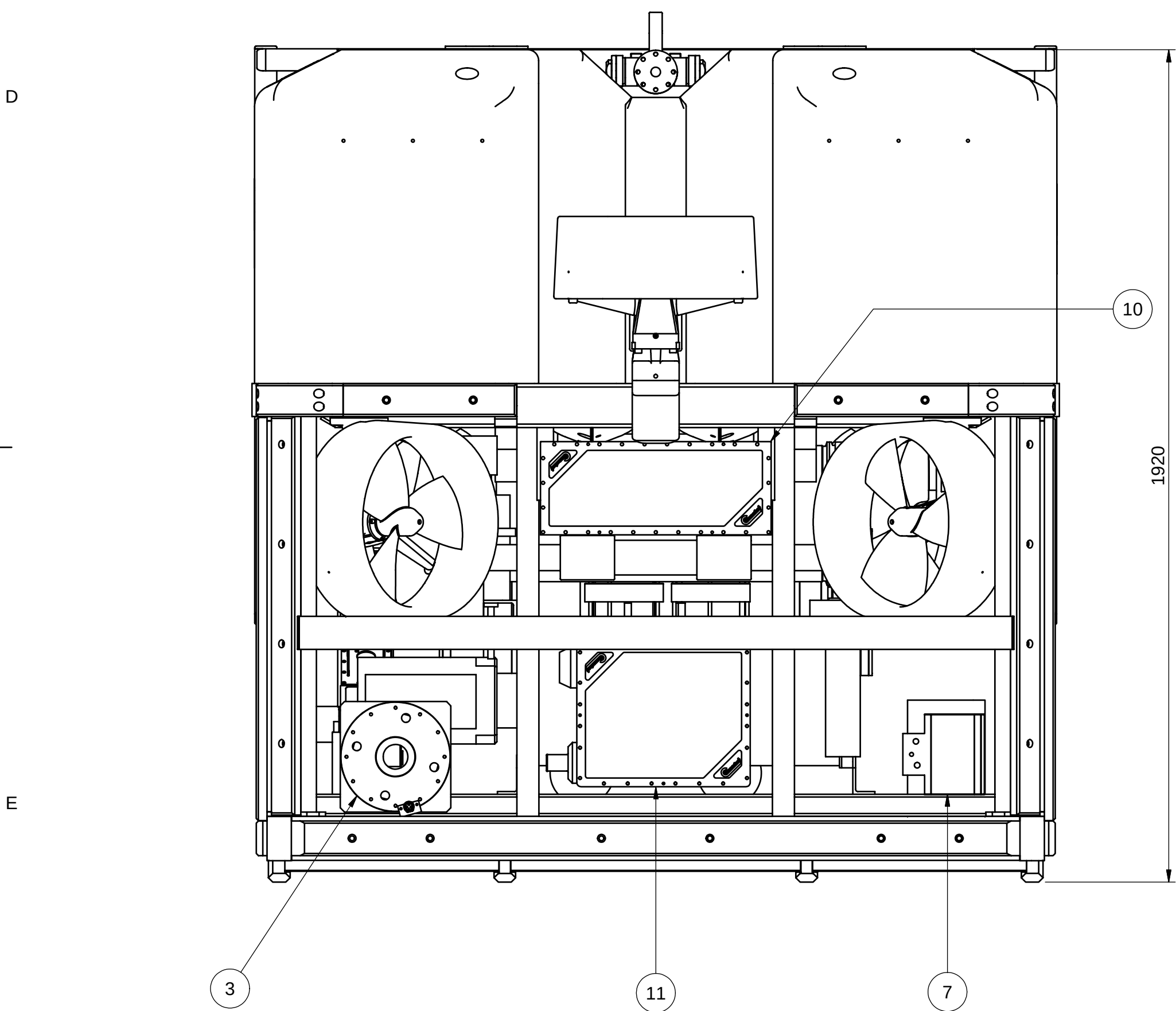
SECTION A-A
