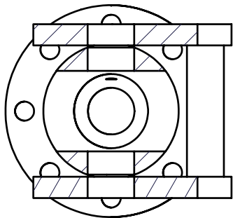
B-B ( 0.40 : 1 )
