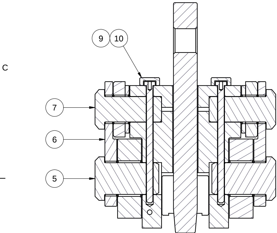
A-A ( 0.40 : 1 )
