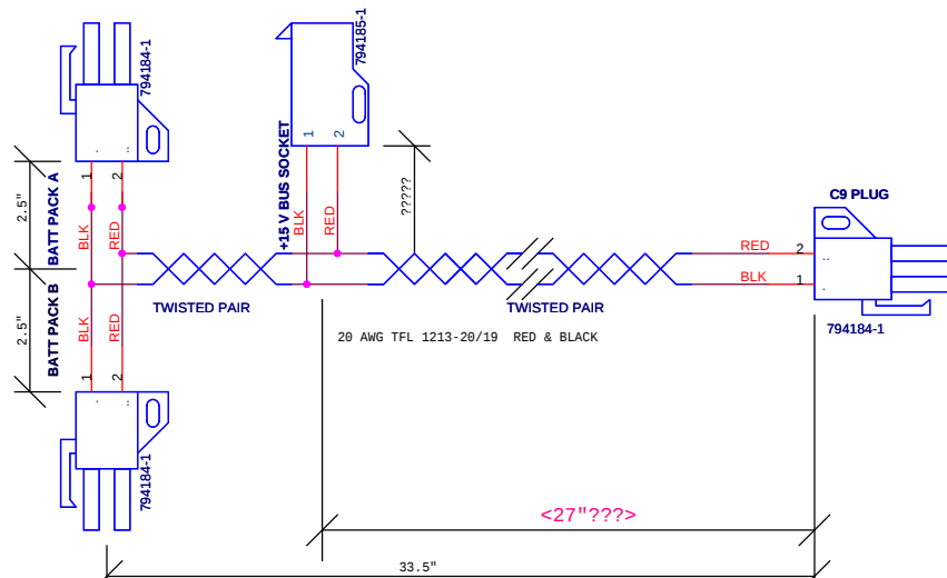
+15 VOLT BATT CABLE
