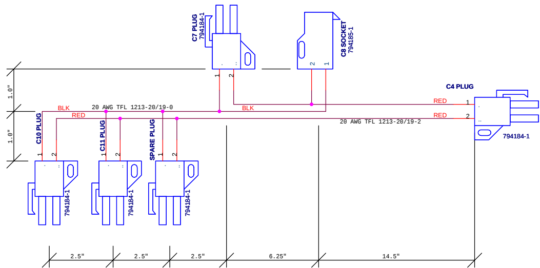
+15 VOLT BUS CABLE
