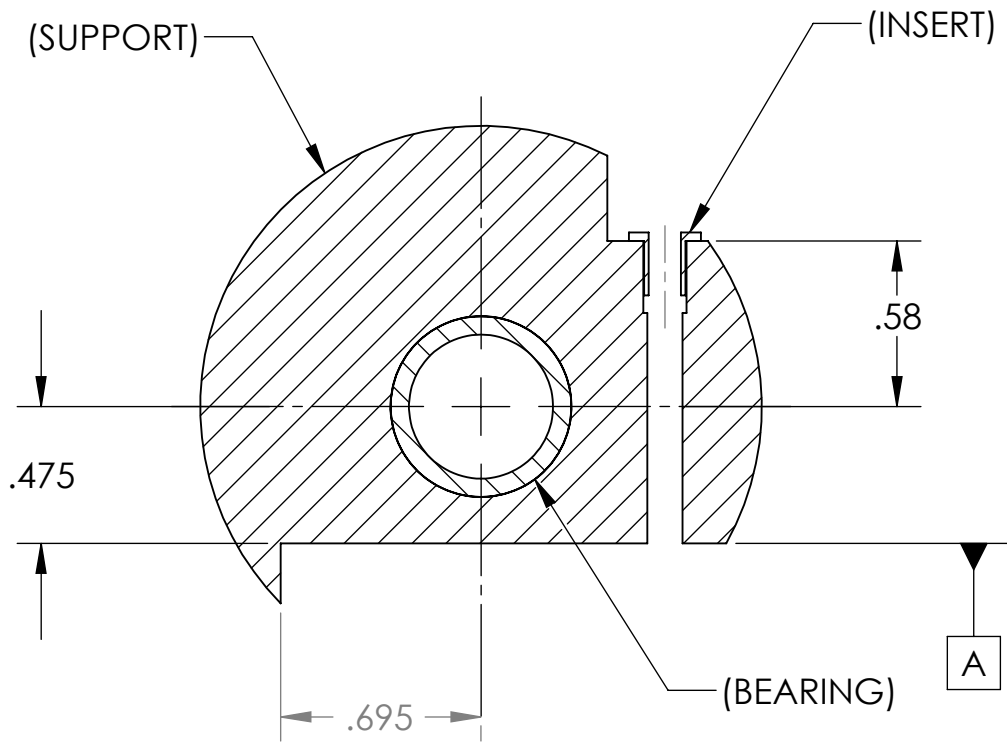
SECTION A-A (01 F5)
