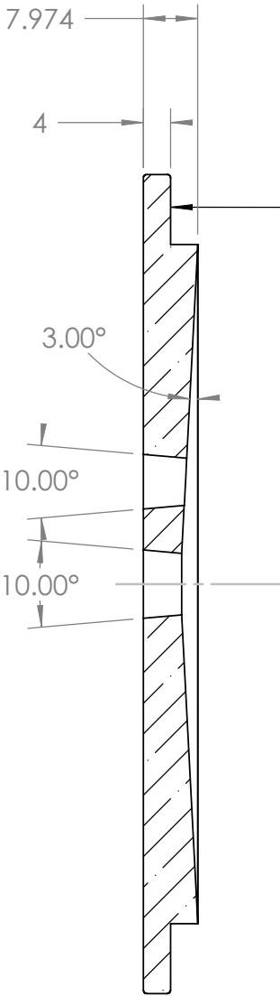
SECTION A-A SCALE 1 : 1
