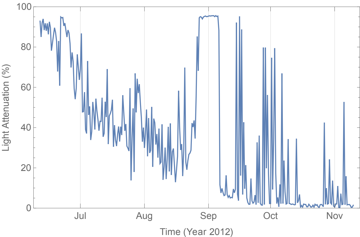
Pulse 60 SES Sediment Quantity
