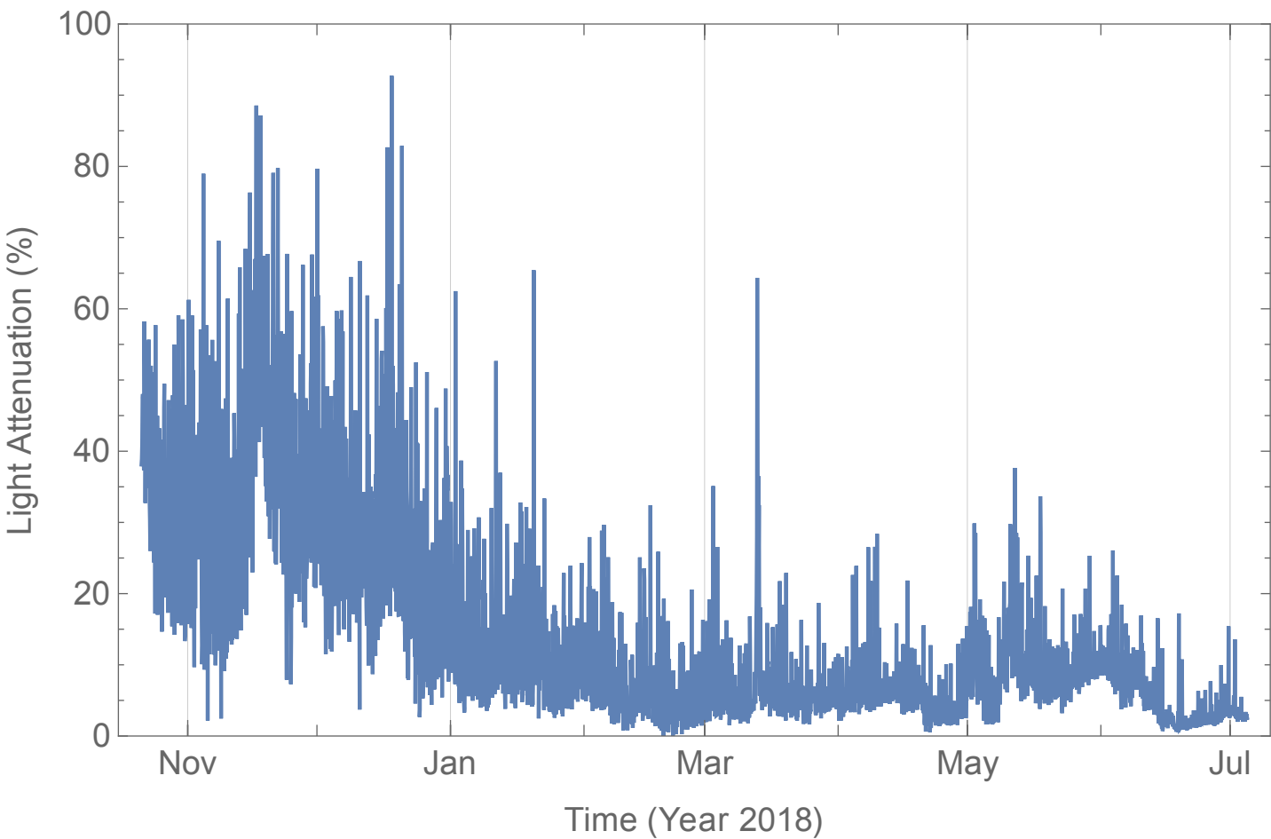
Pulse 71 SES Sediment Quantity
