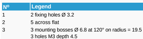
Dimension Diagram : Shaft 79 202 573
