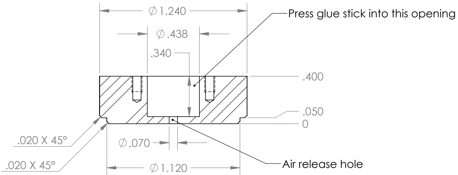
SECTION A-A
