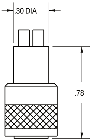
IE55W-10-CCP/UT
