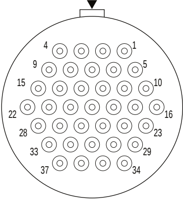
37#16 SCALE 1:1
