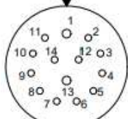
MHDG-14-BCR FACE VIEW
