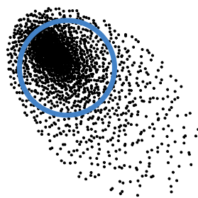
(B): Coma
