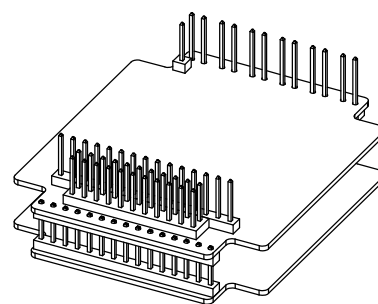
TWE002A,SLDDRW TWE0029A
