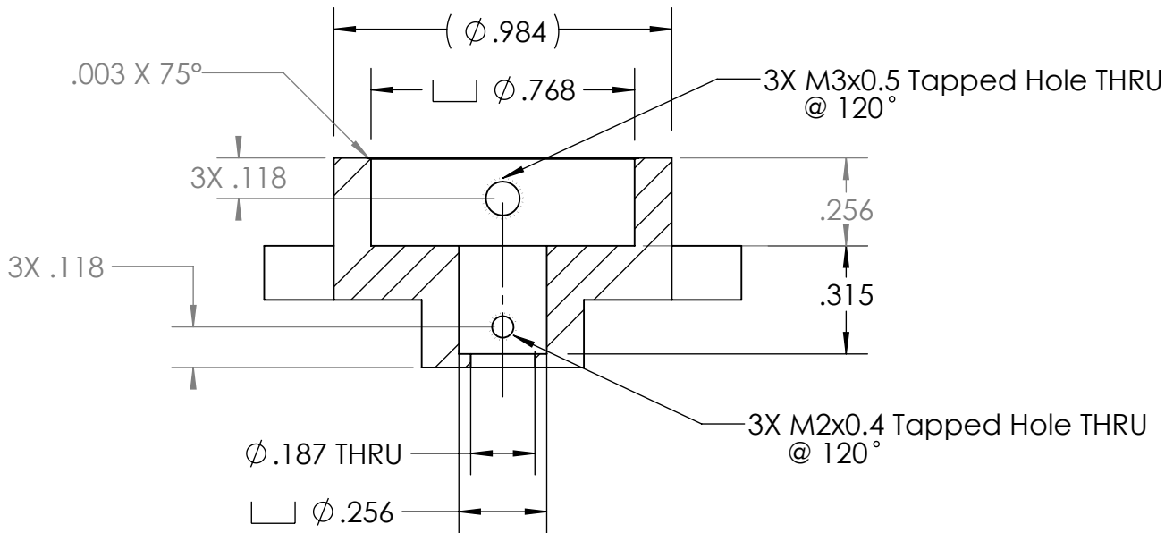
SECTION A-A
