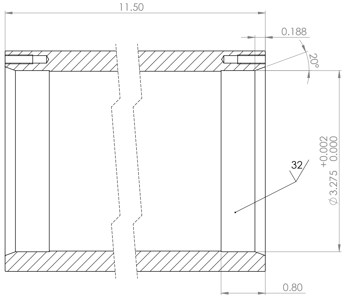
SECTION A-A SCALE 1 : 1
