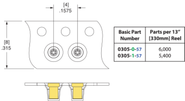
0305-0-57 & 0305-1-57 Tape & Reel Details
