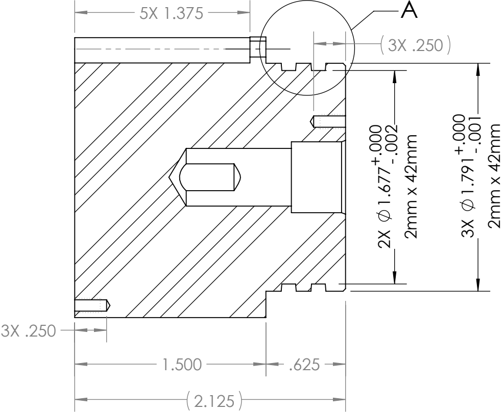
SECTION A-A SCALE 1.3 : 1
