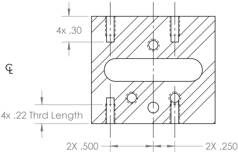
SECTION D-D SCALE 1.5 : 1
