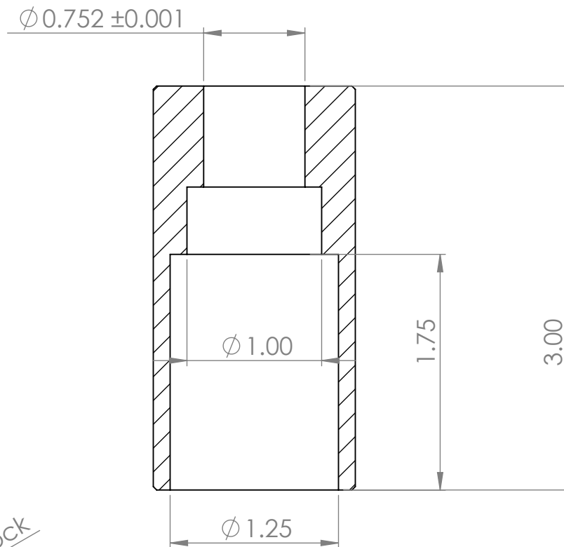
SECTION A-A
