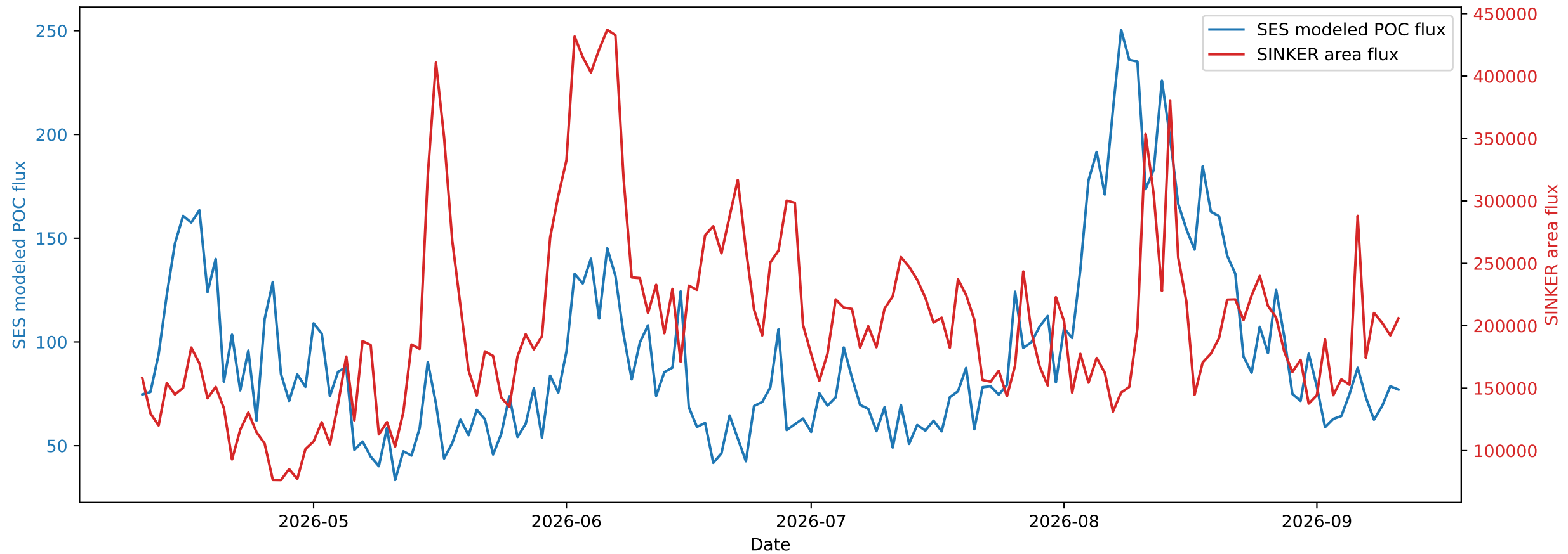
SES and SINKER fluxes
